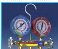
04. VB41332 Servicemanometer 2-veis. Serie 41 for R134a, R404A og R407C
